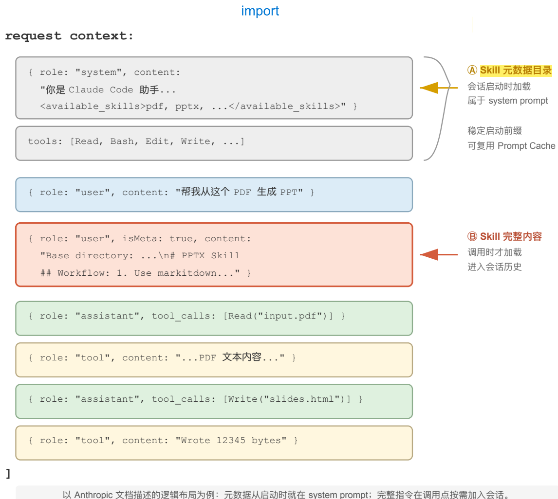
图 2-12 启用 Skills 后 Agent Trajectory 的完整结构
